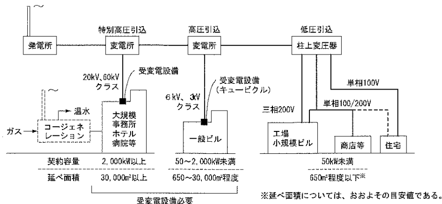
配電方式
