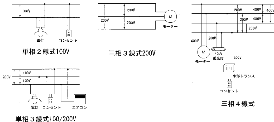
屋内の配線方式の種類
